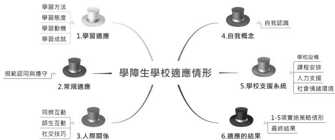
圖 1 研究架構圖
